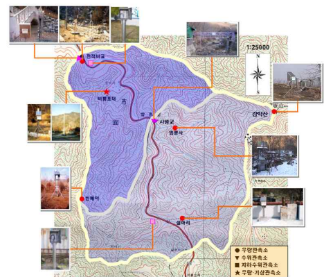
그림 1. 설마천 시험유역도
