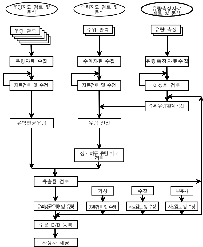
그림 2. 자료처리 흐름도
