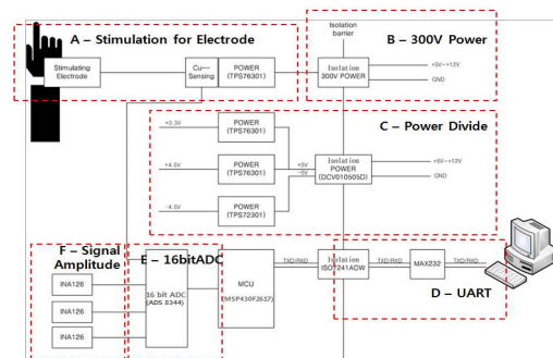
그림 3. 시스템 블록 다이어그램.
