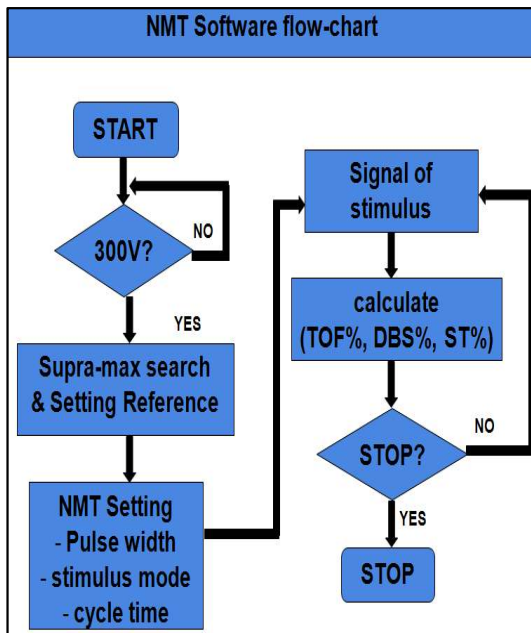
그림 9. S/W 흐름도. Picture 9. S/W Flow Chart.
