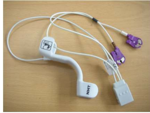
그림 2. MechnoSensor Picture 2. MechnoSensor
