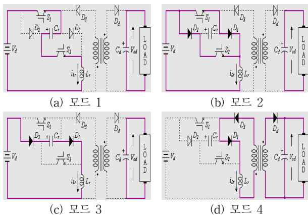
그림 2 스위칭 1주기에 대한 모드별 등가회로 Fig. 2 Equivalent circuits in one cycle switching
