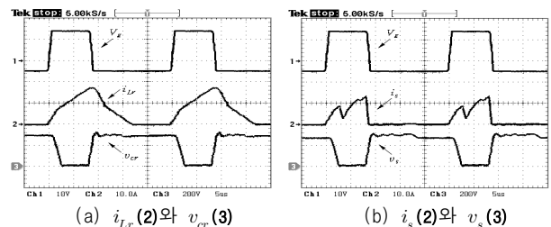
그림 4 스위치 제어신호 V_g 에 대한 각 부의 실험파형 Fig. 4 Experimental waveforms of each part for switching signal
