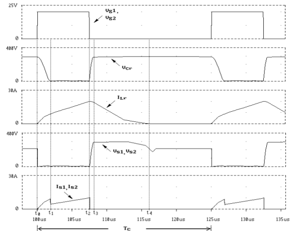
그림 3 스위칭 동작에 의한 시뮬레이션 파형 Fig. 3 Simulation waveforms for switching operation
