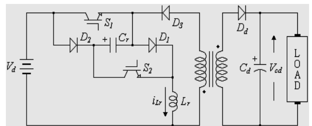
그림 1 제안한 절연형 벡-부스트 컨버터 Fig. 1 A proposed isolated buck-boost converter
