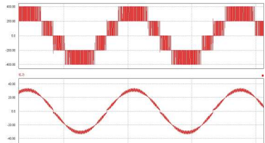
그림 4 인버터 출력 전압과 출력전류 Fig. 4 Output voltage and output current of inverter
