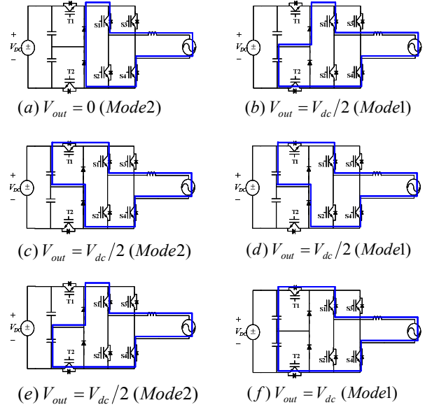
그림 3 양의 반주기 동안의 제안된 인버터의 동작순서 Fig. 3 Operation sequence of proposed inverter in positive half period
