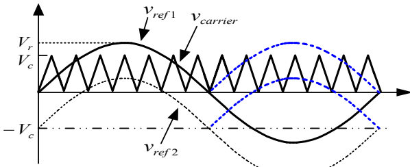
그림 2 반송파와 기준파 파형(0.5 < m a < 1) Fig. 2 Carrier and reference waveforms(0.5 < m a < 1)
