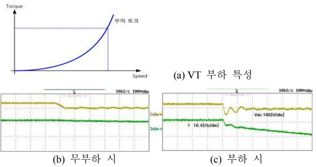
그림 5 부하 특성 및 부하에 따른 Ride-Through 특성
