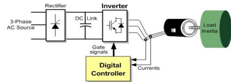
그림 1 유도 전동기 구동 시스템
