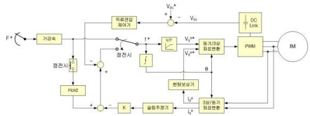
그림 2 Ride-Through 제어 블록
