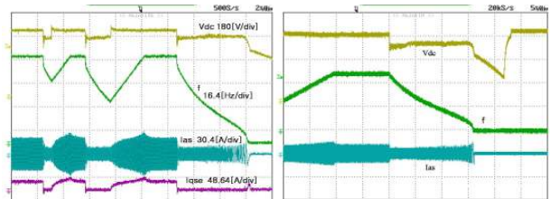
그림 6 슬립 보상 운전
