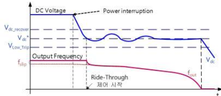
그림 3 Ride-Through 동작
