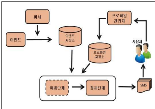
그림 3. 이벤트-프로파일 시스템 구성도
