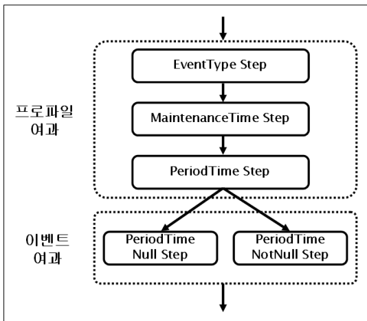
그림 4. 이벤트-프로파일 여과
