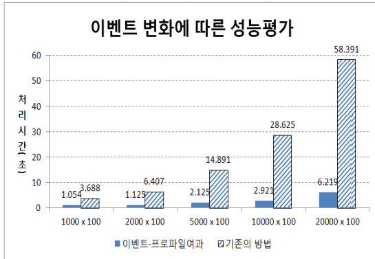
그림 6. 이벤트 변화에 따른 성능평가
