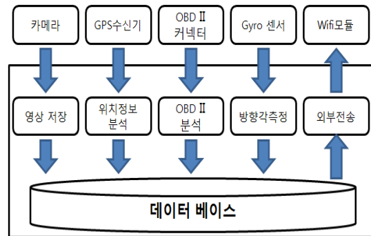
그림 6 프로그램 구성도
