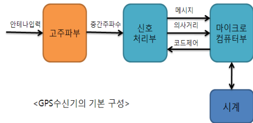
그림 2 GPS수신기의 기본구성도
