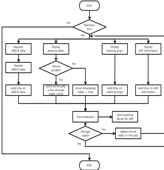
그림 7 시스템 흐름도
