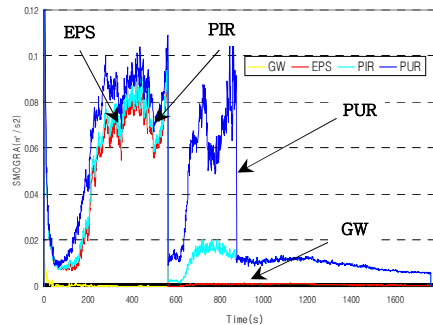
그림 6. SMOGRA 결과 그래프
