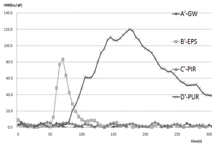
그림 1. ISO 5660-1의 열방출율 결과 그래프
