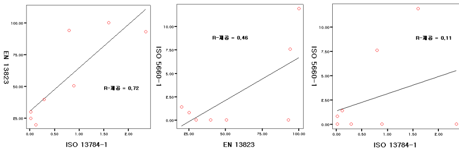
그림 7. 각 규모별 화재시험결과의 상관성 그래프
