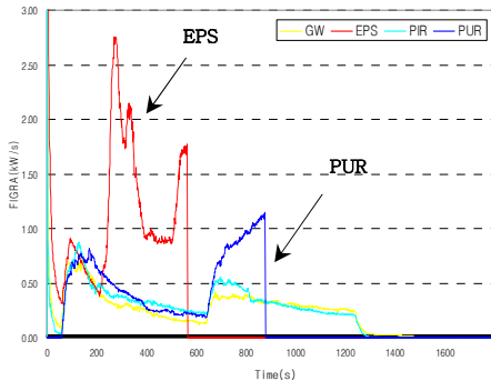
그림 5. FIGRA 결과 그래프
