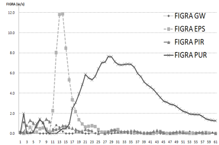
그림 2. ISO 5660-1의 FIGRA 결과 그래프
