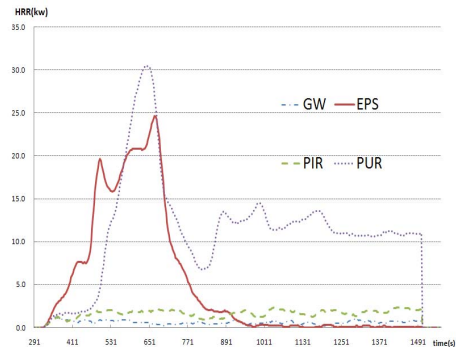
그림 4. EN 13823의 열방출율 결과 그래프
