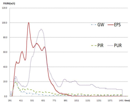
그림 3. EN 13823의 FIGRA 결과 그래프
