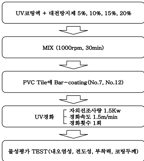
[그림 1] 코팅액 제조 및 UV경화 코팅조건
