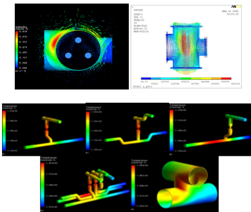
그림 5. CFX(좌측)와 ANSYS(우측)의 속도분포와 와전류 및 온도분포
