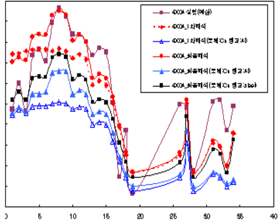
그림 6. 4000A, 5bar(절대압력), 60[Hz] DSES 해석 및 시험결과 비교
