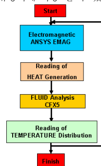
그림 2. 온도상승실험에 사용한 모델
