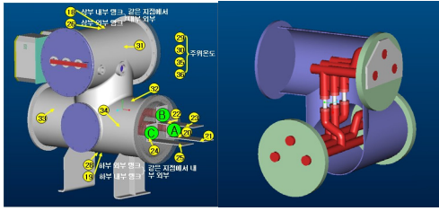
그림 3. 연성해석에 사용되어진 모델
