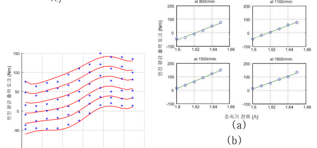
그림 5 디젤 엔진의 운전 조건에 따른 출력 토크 (a) 속도에 따른 토크 (b) 조속기 전류에 따른 토크
