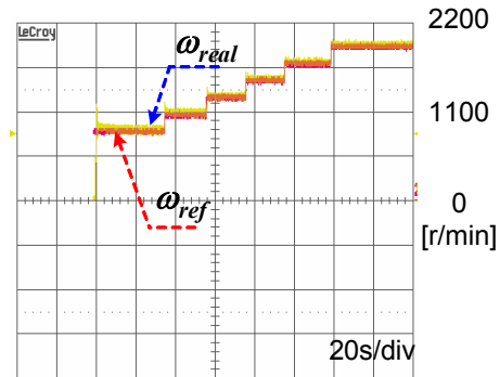
그림 9 K_p = 4, K_i = 0.8, K_d = 0.3 인 경우 전 운전 영역에서의 속도 응답 특성
