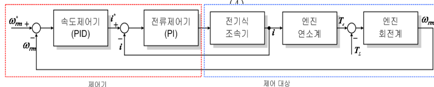
그림 3 전기식 조속기를 이용한 디젤 엔진의 속도 제어 블록 선도
