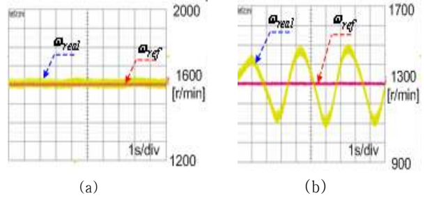
그림 4 K_p = 1, K_i = 0.8, K_d = 0.08 인 경우 디젤 엔진의 속도 응답 (a) \omega_{ref} = 1600 r/min (b) \omega_{ref} = 1300 r/min Fig. 4 Diesel engine speed response for K_p = 1, K_i = 0.8, K_d = 0.08 (a) \omega_{ref} = 1600 r/min (b) \omega_{ref} = 1300 r/min
