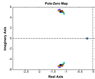
그림 8 K_p = 4, K_i = 0.8, K_d = 0.3 인 경우 공회전으로부터 정격
