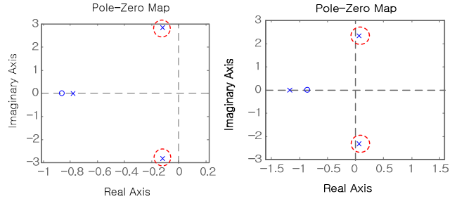
그림 7 K_p = 1, K_i = 0.8, K_d = 0.08 인 경우 식(6)의 극점 영역 점 배치도 (a) \omega_{ref} = 1600 r/min (b) \omega_{ref} = 1300 r/min
