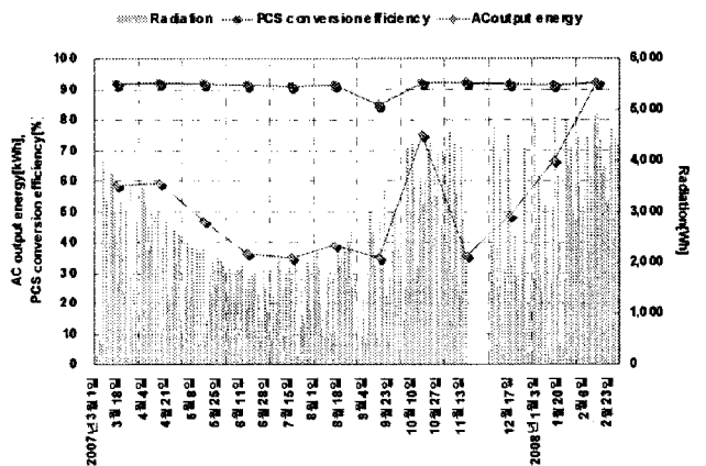
그림 5. 시스템 출력량 및 변환효율
