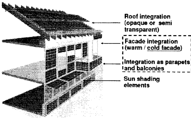
그림 1. 건물일체형 태양광발전시스템 적용 유형
