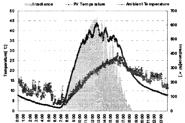
그림 6. PV모듈 후면 및 주변 온도(3월21일)
