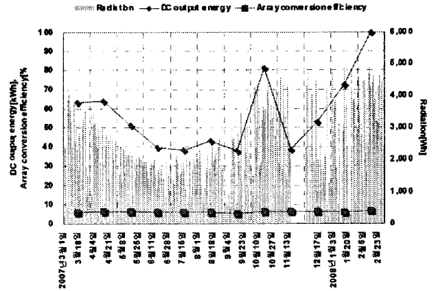
그림 4. PV어레이 출력량 및 변환효율
