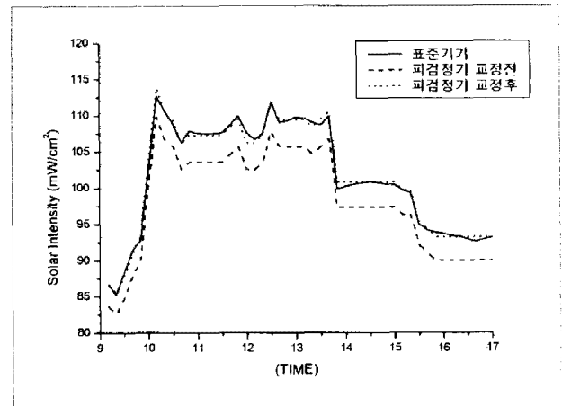
그림 2. 표준기기와의 비교법에 의한 교정 결과
