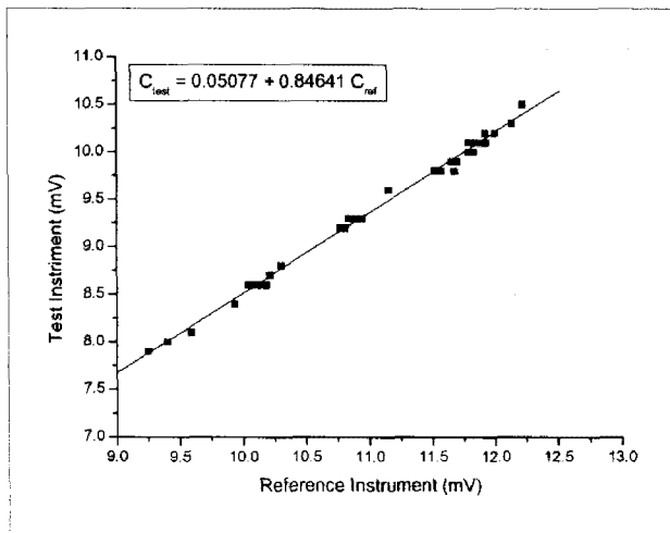
그림 1. 표준기기와의 비교법에 의한 표준기기와 피검정기 출력사이의 상관관계
