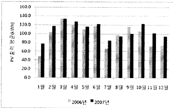
그림 5. 월별 태양전지 출력 평균 전력 특성
