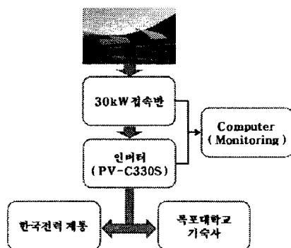
그림 1. 30[kW]급 계통연계형 태양광발전시스템 구성도
