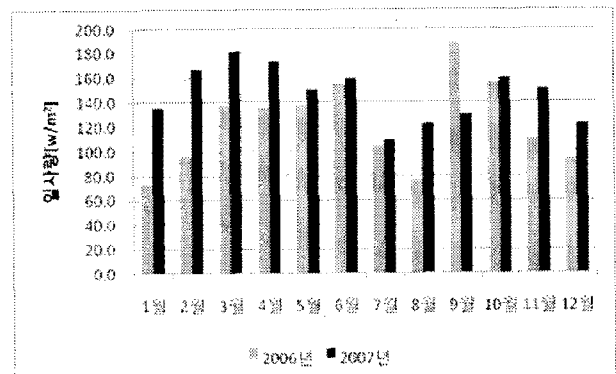
그림 4. 월별 평균 일사량 출력 특성
