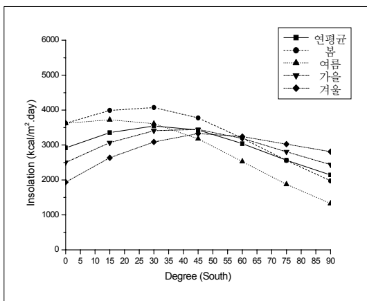
Fig. 3. 남향면에서의 계절별 경사면일사량
