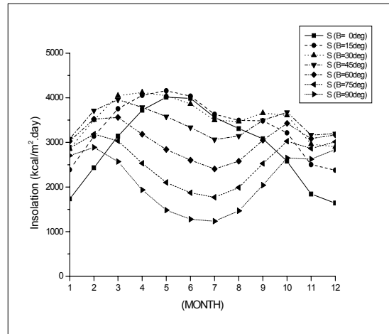
Fig 1. 월별에 따른 남향면 경사면일사량
