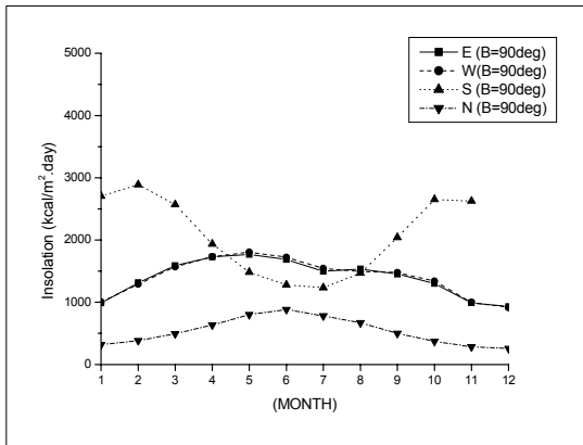
Fig. 2. 월별에 따른 방위별 수직면 경사면일사량
