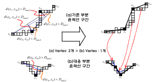
그림 7. 계층적 제어점 매핑 과정
