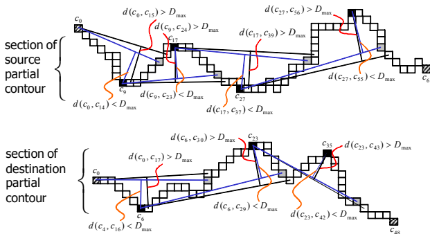
그림 5. 다각형 근사 기반 정점 탐색 과정
