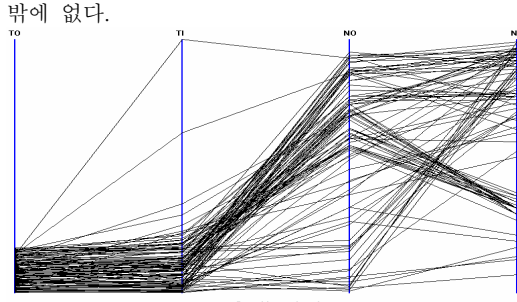
(그림 2) Parallel coordination
