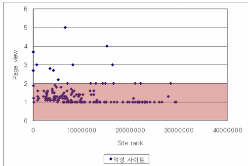
(그림 3) 악성 사이트의 페이지 뷰와 사이트 랭크 분포도
