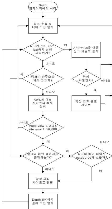
(그림 4) 알려지지 않은 악성 코드 유포 사이트 탐지 기법 순서도
