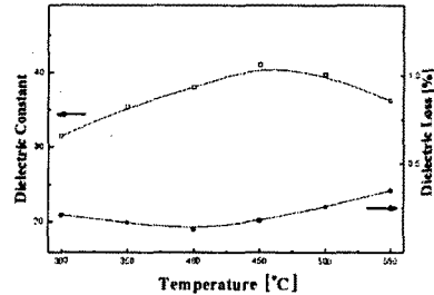
그림 4. 온도에 따른 V_{1.9}W_{0.1}O_5 박막의 유전 특성
