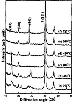
그림 1. 증착 온도에 따른 V_{1.9}W_{0.1}O_5 박막의 XRD 회절모양
