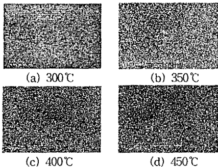
그림 2. 증착 온도에 따른 V_{1.9}W_{0.1}O_5 박막의 단면과 표면 구조
