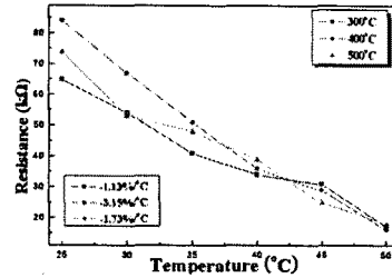
그림 3. 증착 온도에 따른 V_{1.9}W_{0.1}O_5 박막의 TCR값의 변화
