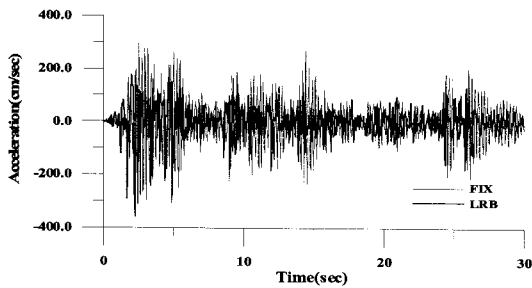
(a) 015-X방향 가속도응답-시간이력
