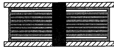
〈그림 3〉 Lead Rubber Bearing
