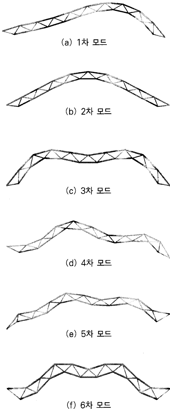
〈그림 7〉 예제 구조물의 진동모드
