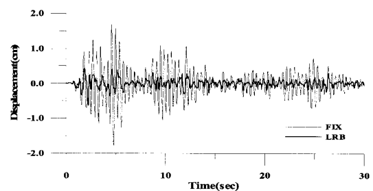
(d) 030-Z방향 변위응답
