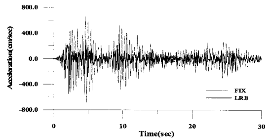
(a) 030-X방향 가속도응답
