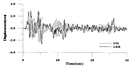
(b) 030-X방향 변위응답
