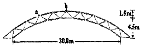
〈그림 6〉 트러스 아치 구조물
