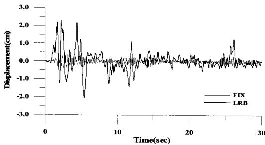
(b) 015-X방향 변위응답-시간이력
