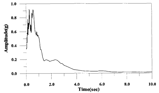
(a) El-Centro NS 가속도스펙트럼
