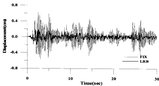
(d) 015-Z방향 변위응답-시간이력
