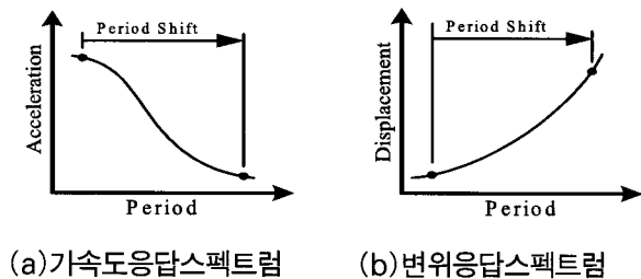
〈그림 2〉 면진시스템에 의한 구조물 거동
