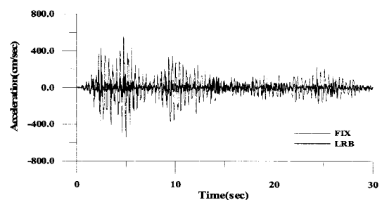
(c) 030-Z방향 가속도응답
