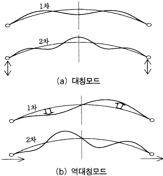
〈그림 1〉 아치구조의 고유진동 모드
