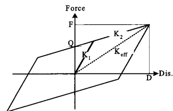
〈그림 4〉 Bilinear 이력거동
