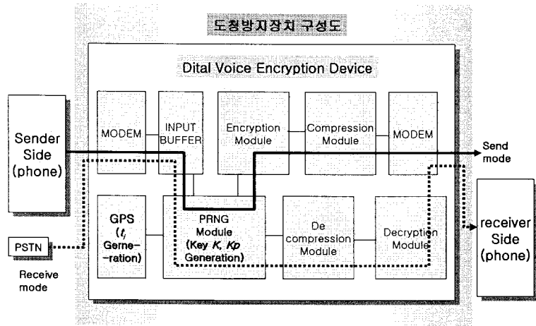
그림 3. 제안하는 도청방지장치 암호화 모듈의 구성도
