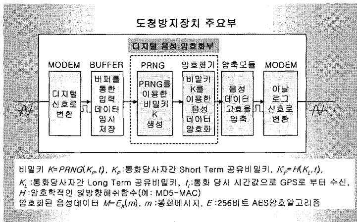
그림 2. 제안하는 도청방지 암호화 모듈
