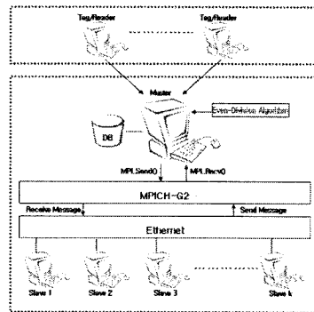
그림 3-3. 그리드 환경의 태그 판별 처리 모델
