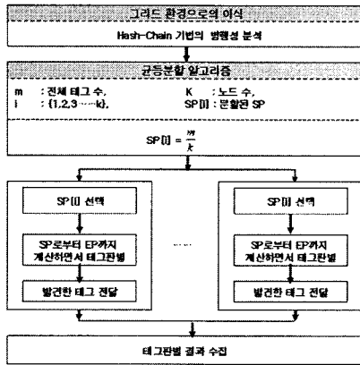
그림 3-5 균등분할 알고리즘을 이용한 태그 판별 처리 흐름도
