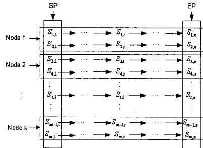
그림 3-2. 동일한 크기에 따른 균등분할 알고리즘
