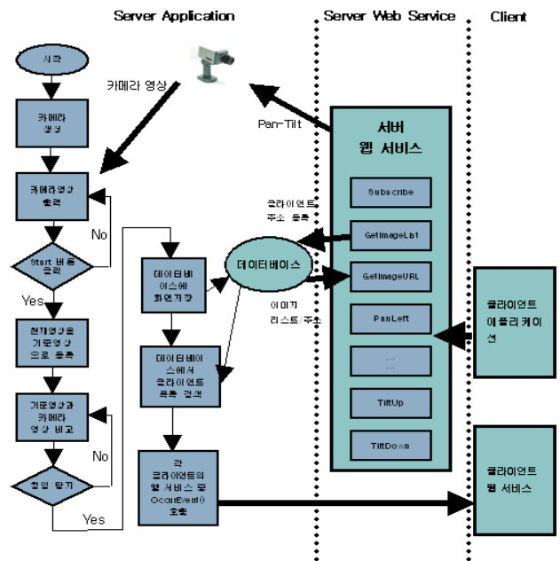
(그림5) 서버 시스템의 실행 흐름도
