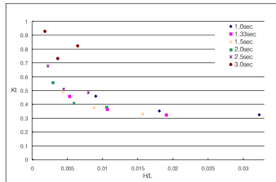
Fig. 4. 전달율
