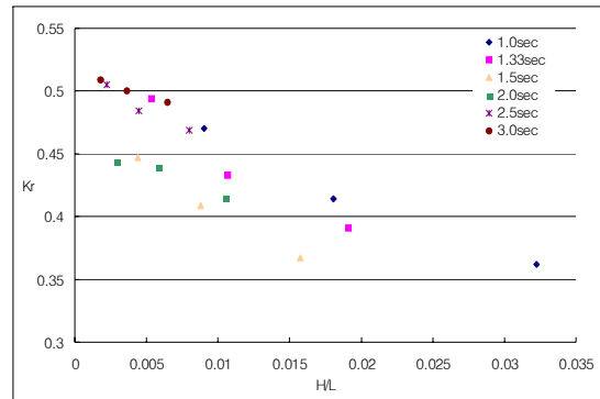
Fig. 3. 반사율
