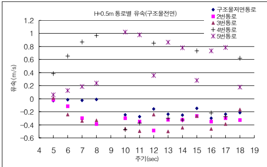
Fig. 5. 구조물 전면유속
