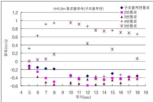
Fig. 6. 구조물 후면 유속
