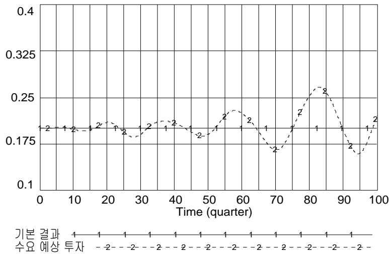
<그림 3-12> 수요 예상 투자에 의한 시장점유율 추이의 변화(수요 정체 시)
