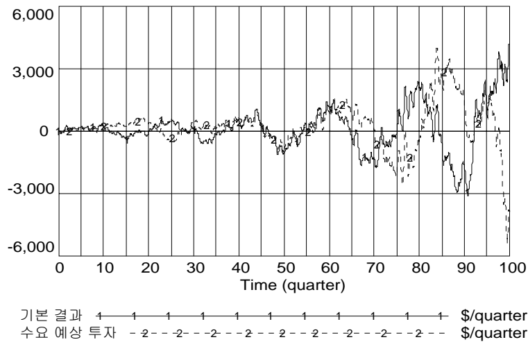
<그림 3-24> 수요 예상 투자에 의한 순수익 추이의 변화(수요 성장 시)
