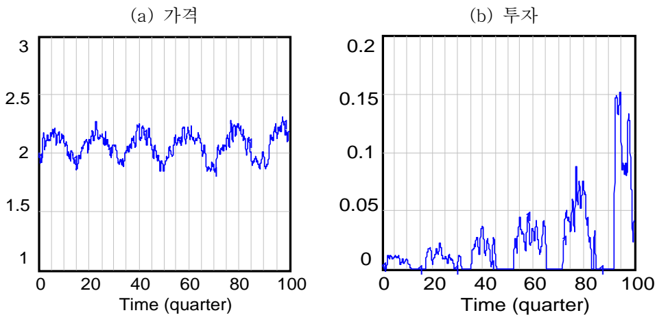
<그림 2-8> 가격과 투자의 추이(수요 성장의 경우)
