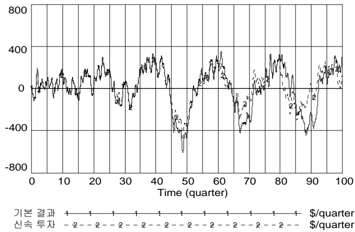
<그림 3-5> 설비구축기간 단축에 따른 순수익 추이의 변화(수요 정체 시)
