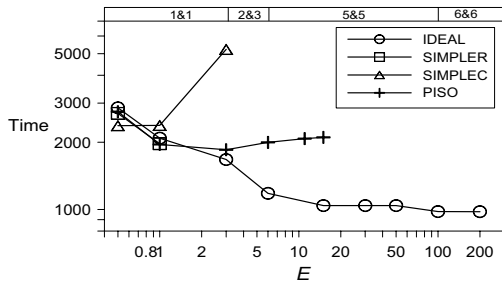
(b) Re=500
