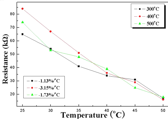
〈그림 3〉 증착온도에 따른 V_{1.8}W_{0.2}O_5 박막의 TCR값의 변화
