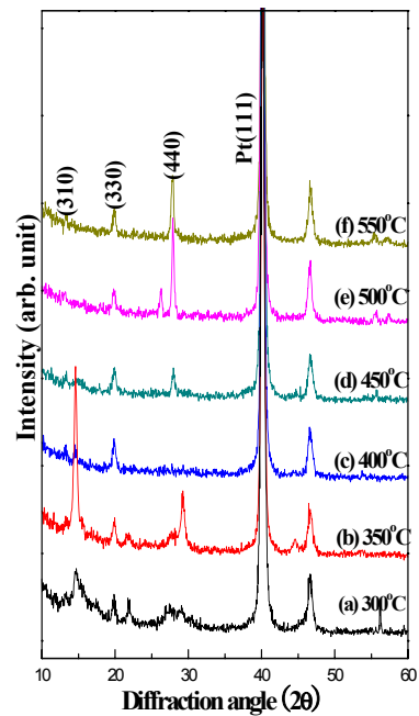
<그림 1> 증착온도에 따른 V_{1.8}W_{0.2}O_5 박막의 XRD 회절모양
