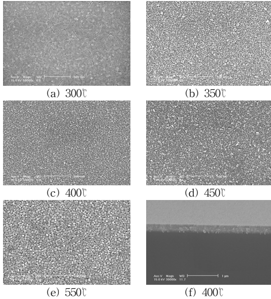
〈그림 2〉 증착온도에 따른 V_{1.8}W_{0.2}O_5 박막의 단면과 표면 구조
