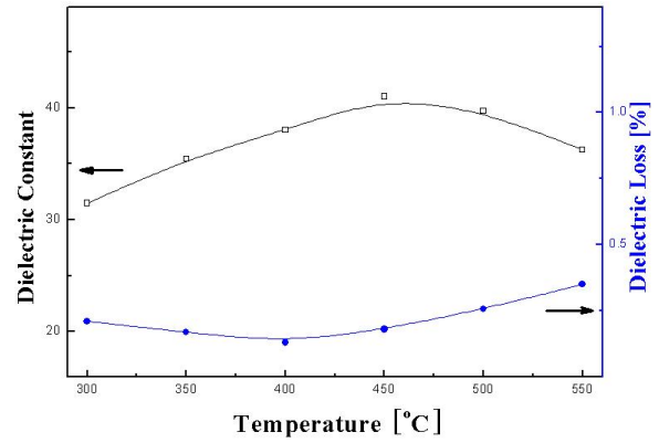
〈그림 4〉 온도에 따른 V_{1.8}W_{0.2}O_5 박막의 유전 특성
