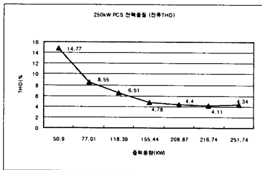
Fig 8. 250kW PCS 전력품질곡선(전류THD)
