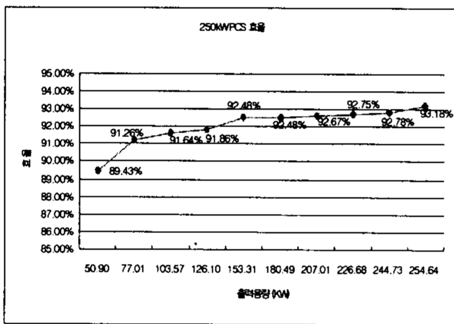
Fig 7. 250kW PCS의 전부하 효율곡선
