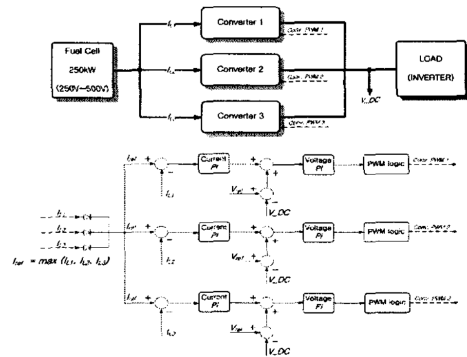
Fig 3. DC-DC 컨버터 제어블럭도
