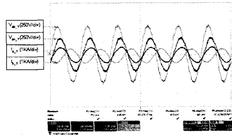
(d) 250kW 정격부하 운전(계통연계제어)
