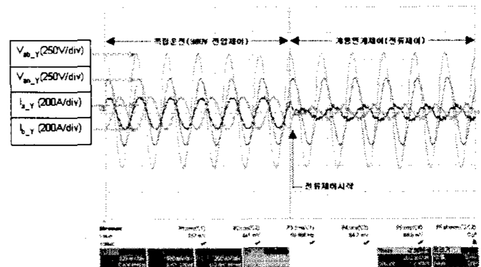
(c) 전압제어에서 전류제어모드로 전환
