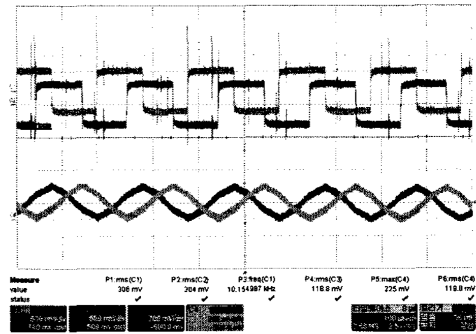
(a) DC-DC 컨버터 스위칭 및 인덕터 전류파형
