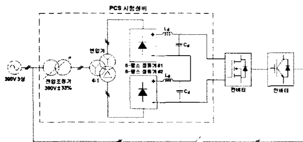
Fig 5. 250kW급 PCS 시험설비
