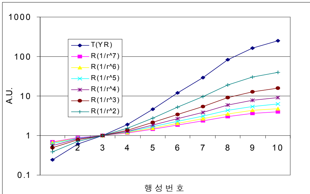
그림3 중력 승수에 따른, 공전주기에서 환산한 태양-행성간 거리의 변화
