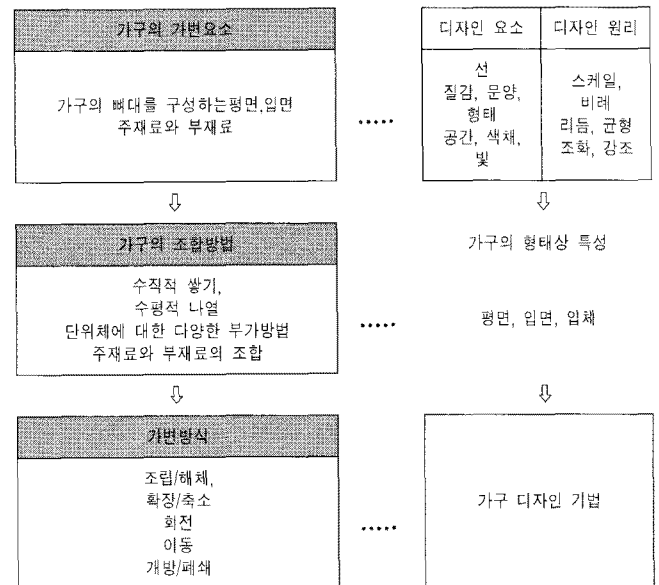
<표 3> 디자인요소와 원리에 따른 가변가구의 디자인기법
