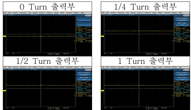
〈그림 8〉 단자 이완 검출 장치 최종 출력 파형
