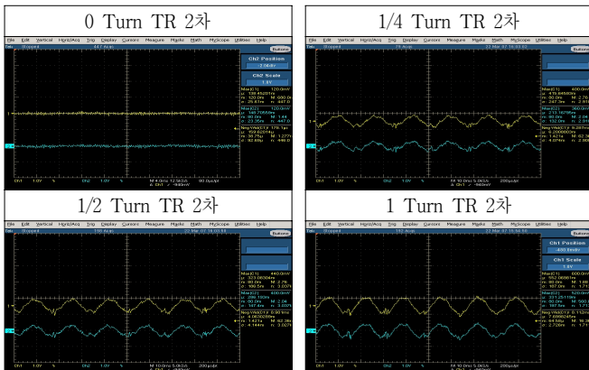
〈그림 5〉 TR 2차 유기 전압 파형
