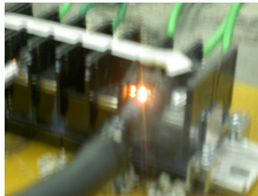
<그림 2> 단자대 접촉 불량 발화 상태
