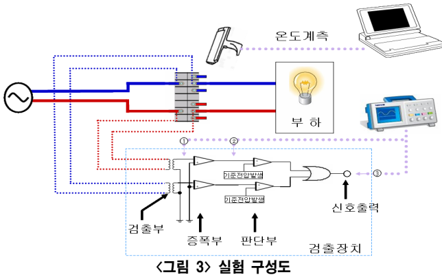
〈그림 3〉 실험 구성도
