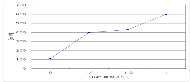
〈그림 6〉 TR 2차 유기 전압 파형 크기 변화 그래프
