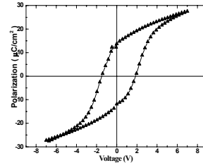
〈그림 4〉 PZT(10/20/10) 다층 박막의 이력곡선
