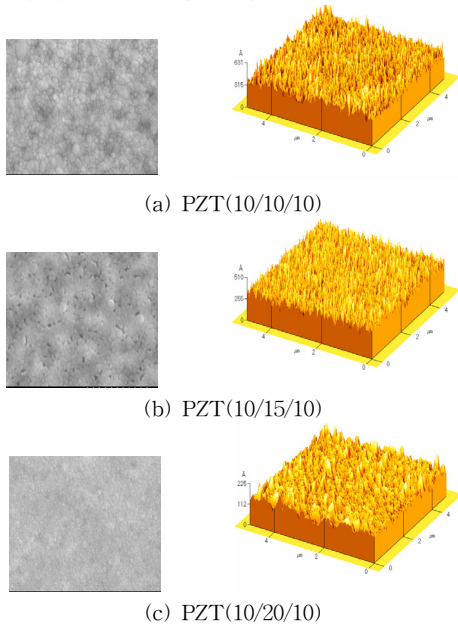
〈그림 2〉 PZT(6040) 박막 두께에 따른 PZT 다층 박막의 AFM과 표면 구조
