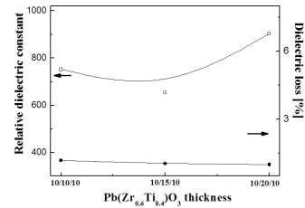
〈그림 3〉 PZT(6040) 박막 두께에 따른 PZT 다층 박막의 유전특성
