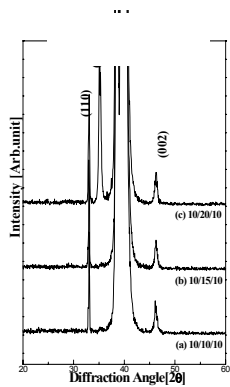
〈그림 1〉 PZT(6040) 박막 두께에 따른 PZT 다층 박막 XRD 회절 패턴
