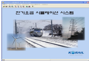
그림 2 GUI 메인화면
