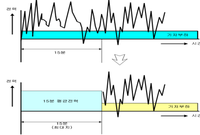
그림 1 기본전기요금 개념
