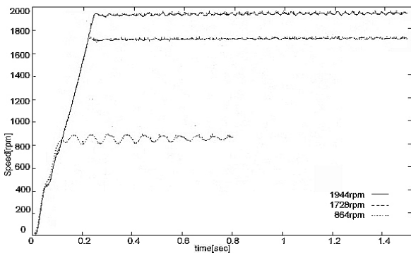
〈그림 3〉 속도 응답
