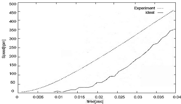
〈그림 2〉 가속 시 속도 응답(3000rpm) 확대
