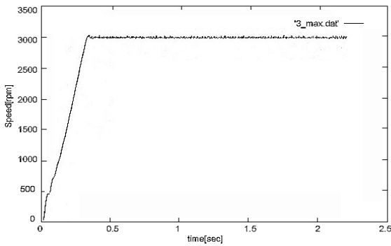
〈그림 1〉 속도 응답(3000rpm)
