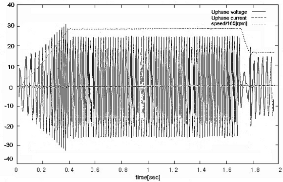
〈그림 4〉 감속 시에 전압, 전류파형
