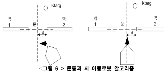
<그림 6 > 문통과 시 이동로봇 알고리즘
