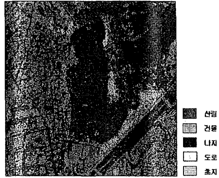
그림 6. K-means
