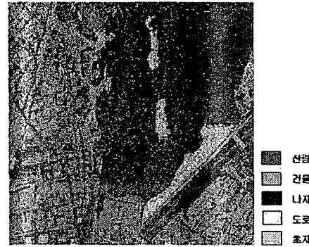
그림 7. Neural Network
