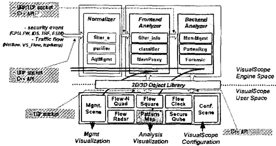
[그림 5] VisualScope의 구조
