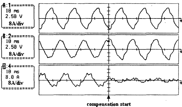
그림 10 가상부하기와 전력회수기 출력전류, 그리고 전원전류 Fig. 10 Dummy load unit output current, power recovery unit output current and source current
