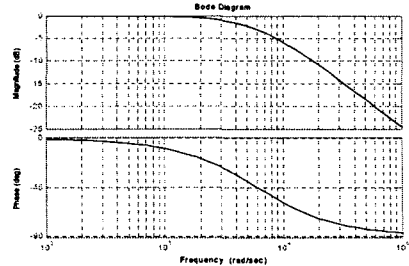
그림 4 bandwidth=6000[rad/sec]일 때 전달함수의 bode선도 Fig. 4 Bode diagram of transfer function at bandwidth = 6000[rad/sec]
