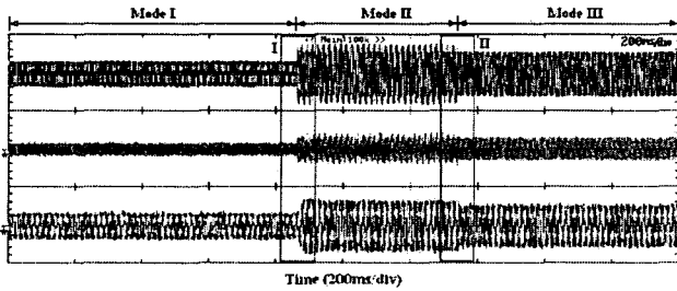
(a) 부하전류, 보상전류, 그리고 전원전류(12A/div) (a) Load current, compensating current and source current
