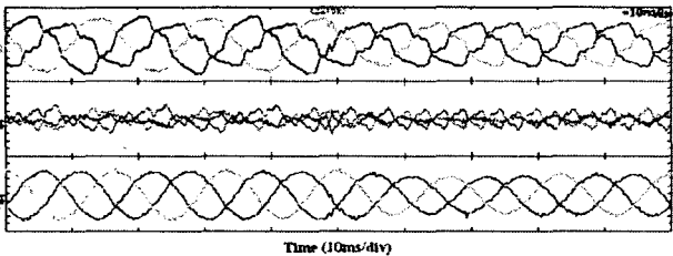
(c) 영역II의 확대파형(12A/div) (c) Expanded waveform of region II 그림 9 부하 모드 I, II, III에 대한 실험파형 Fig. 9 Experimental results for load mode I, II and III
