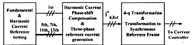
그림 5 고조파 위상지연 보상 Fig. 5 Configuration of harmonic phase-delay compensation
