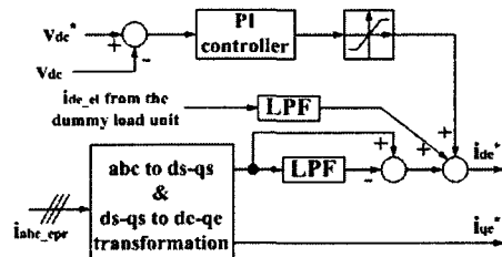
그림 6 전력회수기의 기준전류 생성 Fig. 6 Current reference extraction of the power recovery unit
