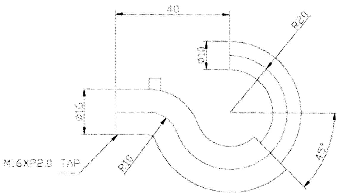
그림 6. 전주 보호용 기구 개략도 Fig. 6. Outline of Tool for Protection of Electric Pole
