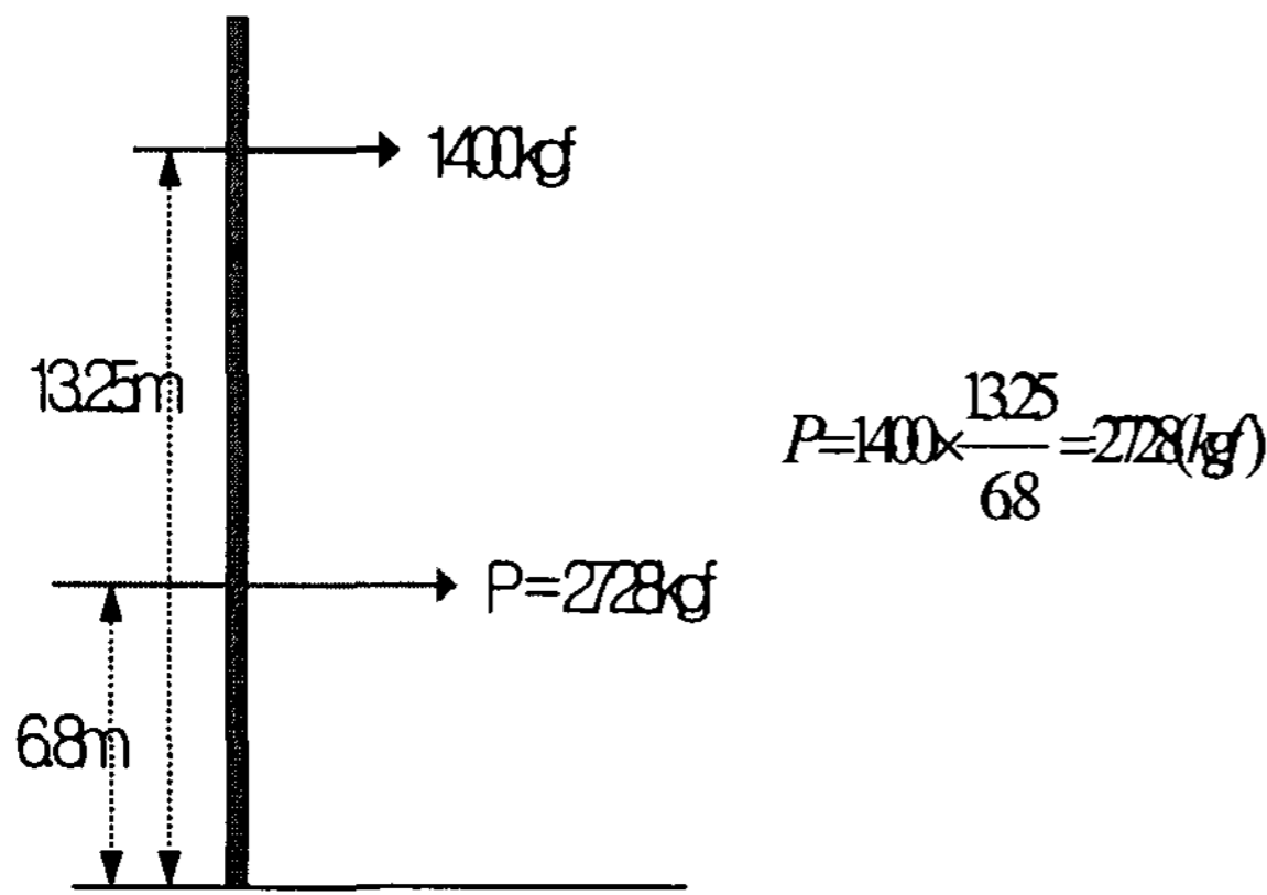
그림 2. 굽힘 모멘트에 대한 파괴 하중 Fig. 2. Breakdown Load for Bending Moment
