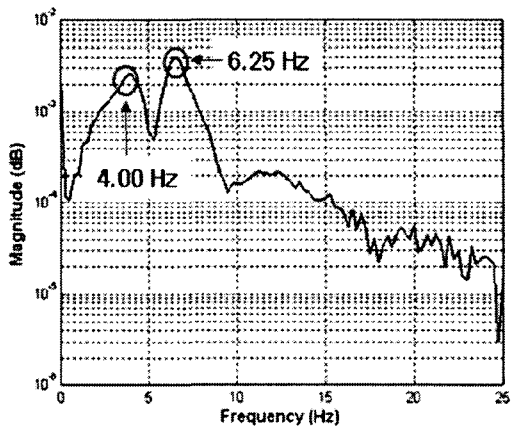
(b) Power spectrum (z-dir)
