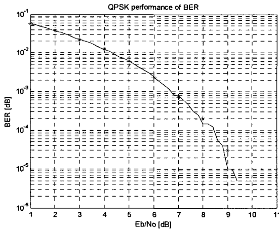
그림 9 AWGN 채널에서 QPSK 의 BER 특성
