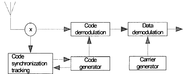
그림 5 DS-SS 수신기의 블록도
