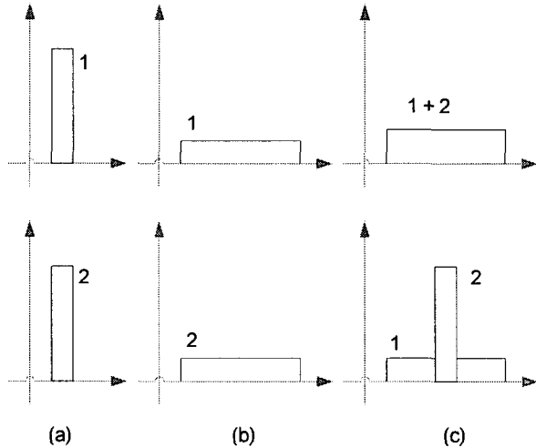
그림 1 확산 역확산 원리
