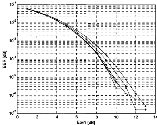
그림 8 센서 증가에 따른 BER 특성
