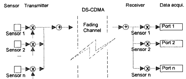
그림 7 DS-CDMA를 이용한 다중 센서 데이터 전송
