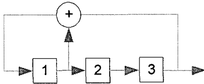
그림 6 3 상태 M 시퀀스의 LSR
