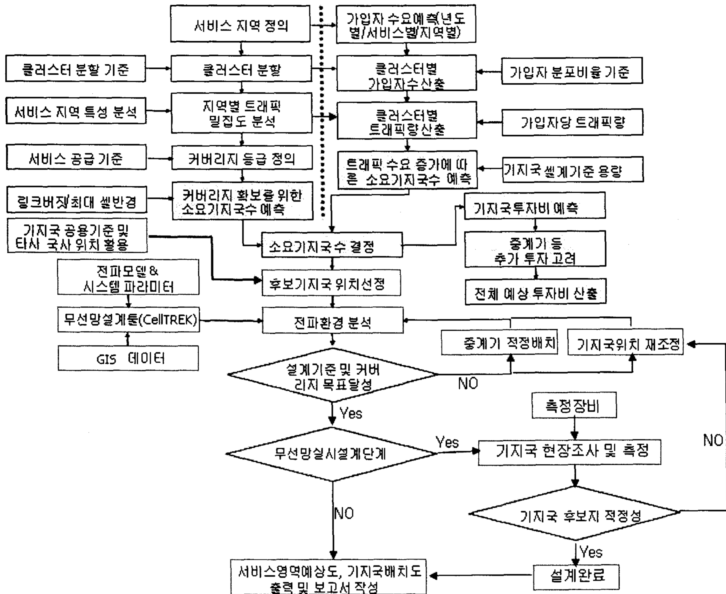
그림 1. 무선망 설계절차
