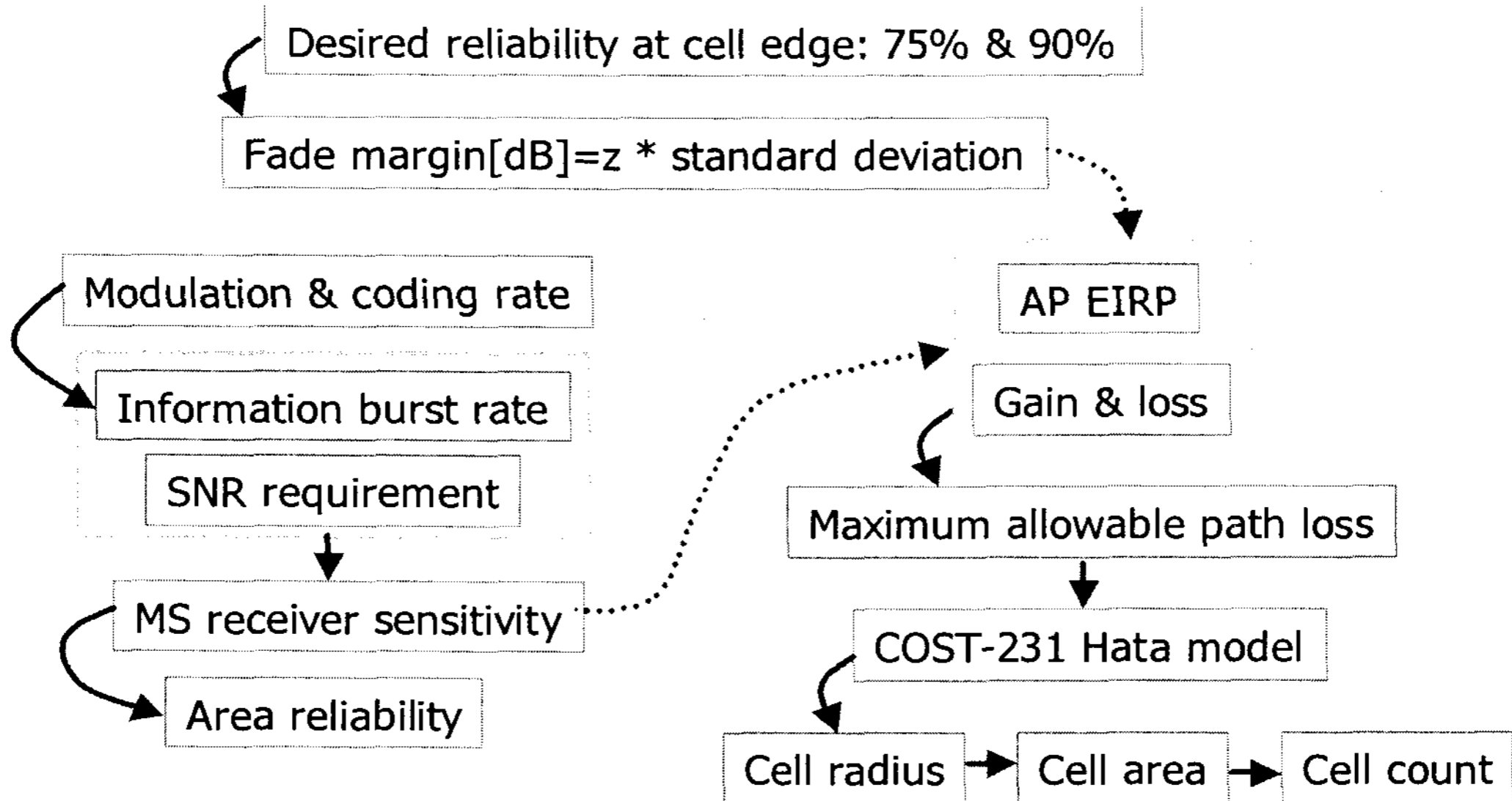
그림 3. 셀 반경 및 면적 계산 방법
