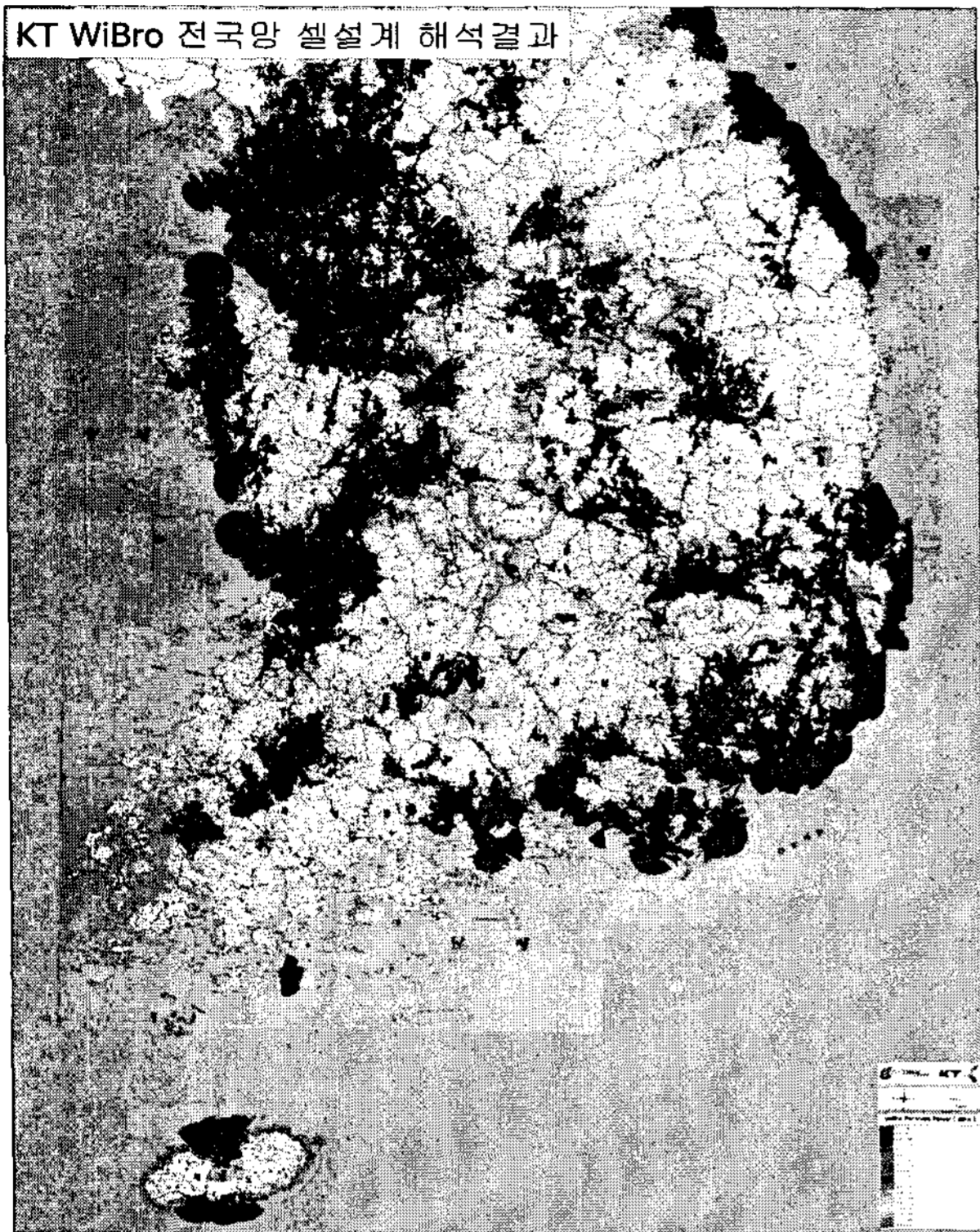
그림 5. KT WiBro 전국망설계 결과
