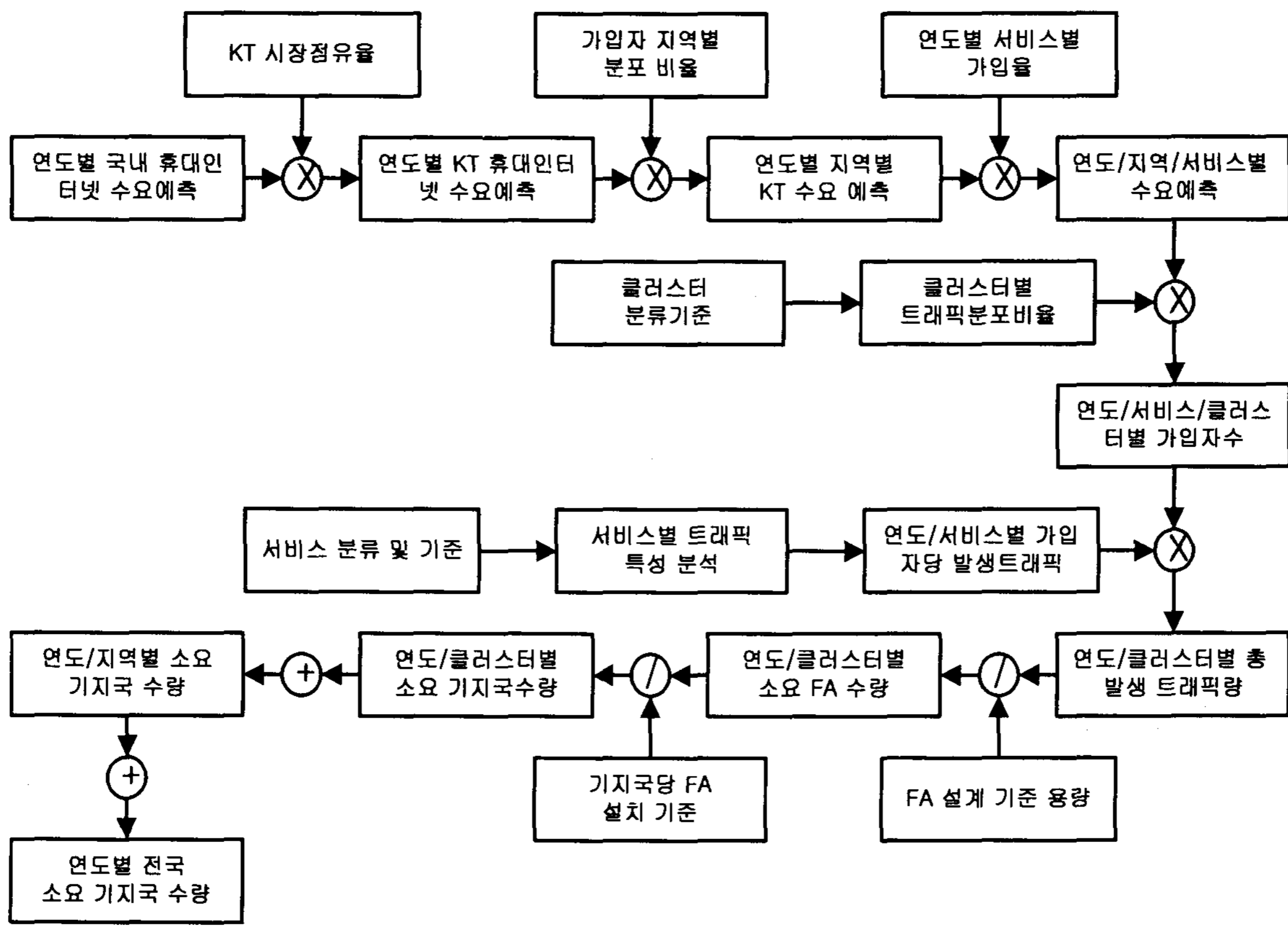
그림 4. 트래픽에 의한 기지국 수량 산출 흐름도
