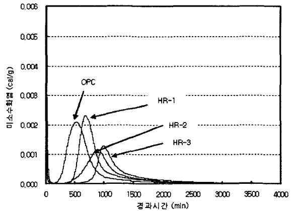
그림 2. 수화열 저감제/용매비에 따른 미소수화열 변화
