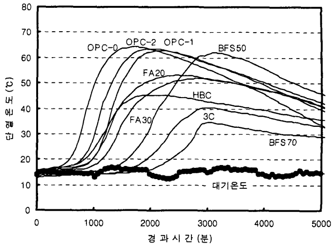
그림 4. 결합재 종류에 따른 간이 단열온도 측정 결과
