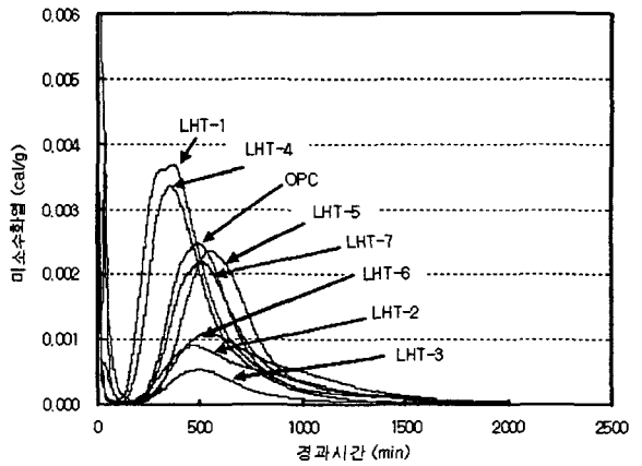
그림 1. 수화열저감제 종류에 따른 미소수화열 변화
