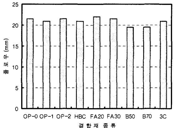
그림 3. 결합재 종류에 따른 모르타르 플로우 변화
