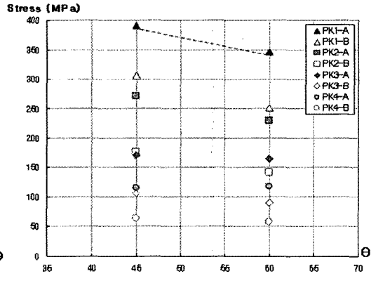
(b) \theta 에 따른 Brace heel의 응력
