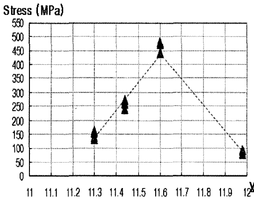
(a) \gamma 에 따른 Chord heel의 응력
