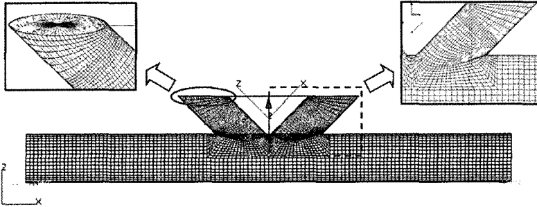
그림 3 모델링
