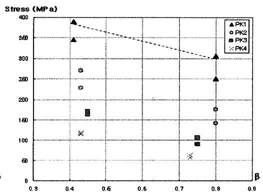
(b) \beta 에 따른 Brace heel의 응력
