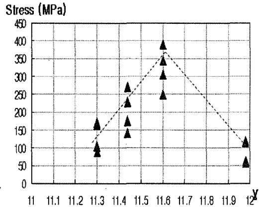
(b) \gamma 에 따른 Brace heel의 응력
