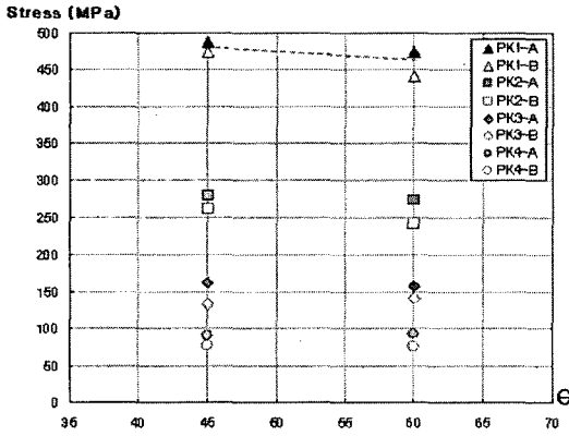
(a) \theta 에 따른 Chord heel의 응력
