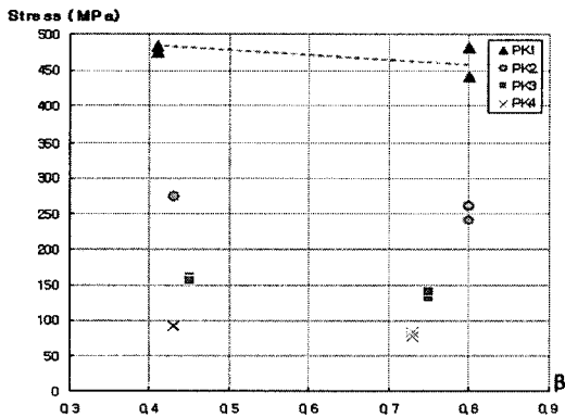
(a) \beta 에 따른 Chord heel의 응력
