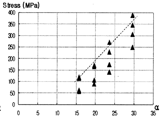
(b) Brace heel의 응력
