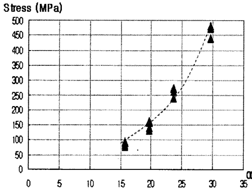
(a) Chord heel의 응력
