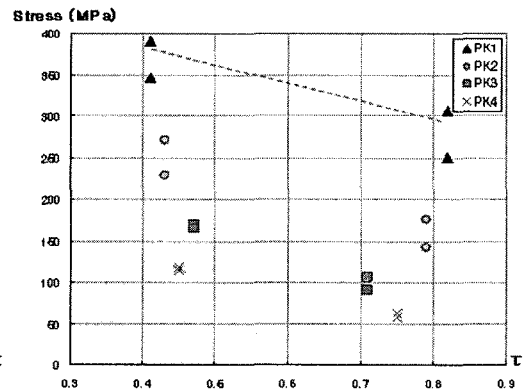
(b) \tau 에 따른 Brace heel의 응력
