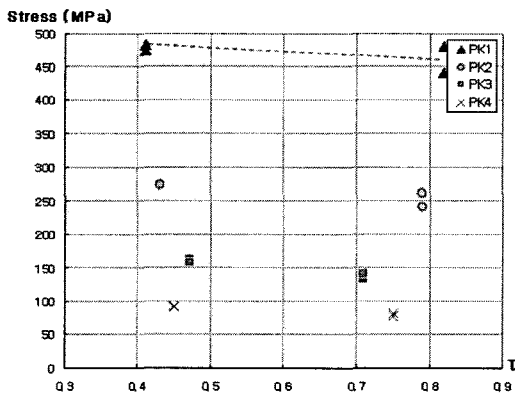
(a) \tau 에 따른 Chord heel의 응력
