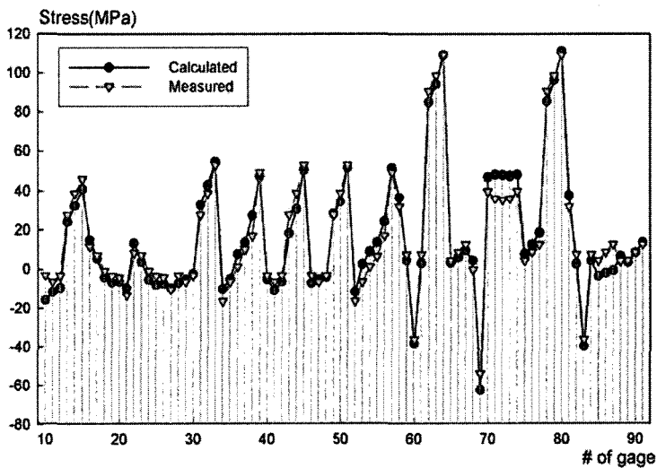
그림 2 실험값/해석값 비교
