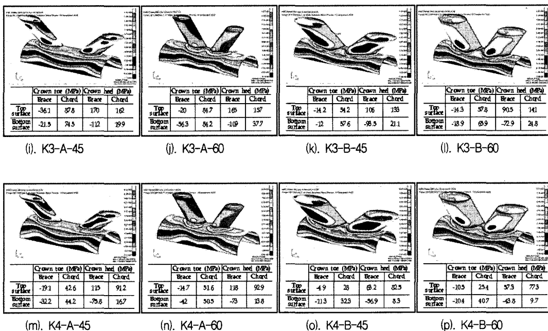
그림 4 수치해석 결과정리
