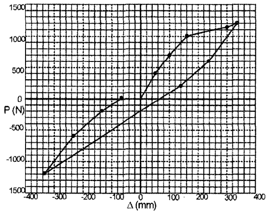
그림 3. 예제구조물 하중-변위도
