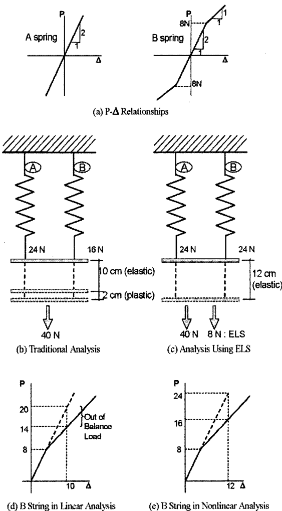
그림 1. 단자유도 비선형 구조물의 강성등가하중
