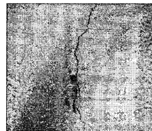
사진 5. 노출표면의 소성 수축 균열
