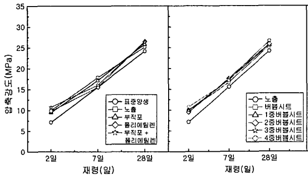
그림 3. 표면양생방법별 압축강도 특성
