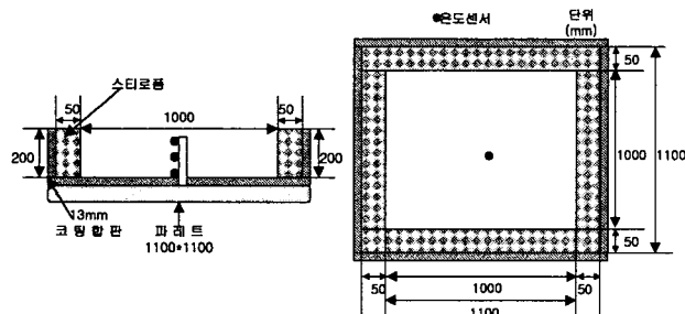
그림 1. 모의 시험체 평·단면도
