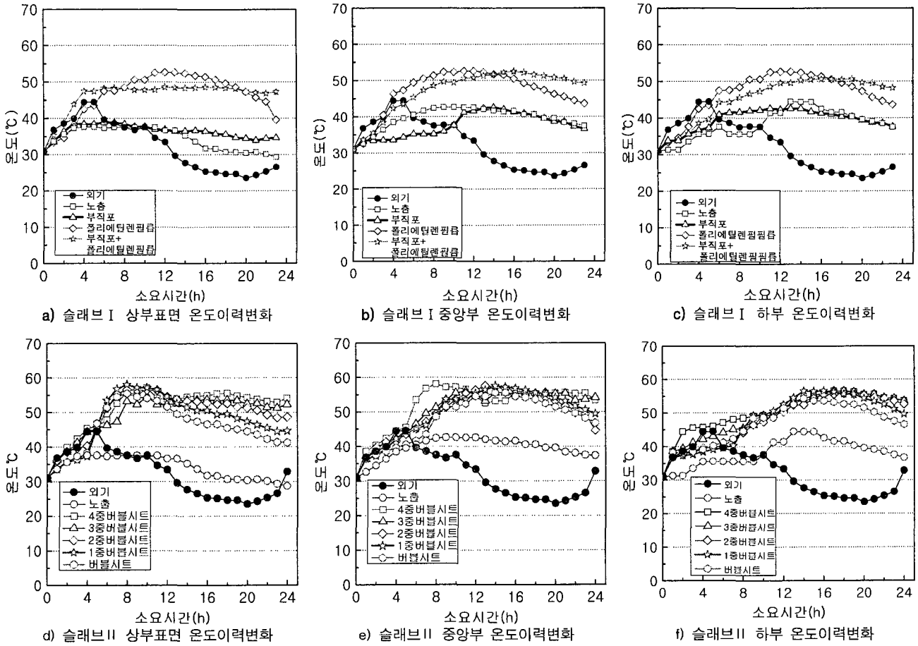
그림 2. 표면양생 방법별 슬래브의 온도이력
