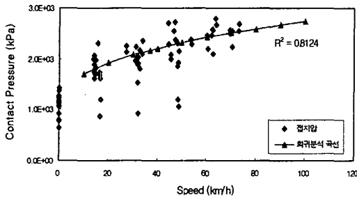
그림 4. 차량속도에 따른 동적 점지압
