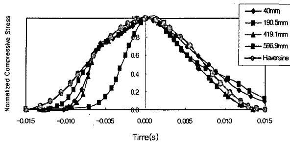
그림 2. FWD하중에 의한 깊이별 하중지속시간의 변화
