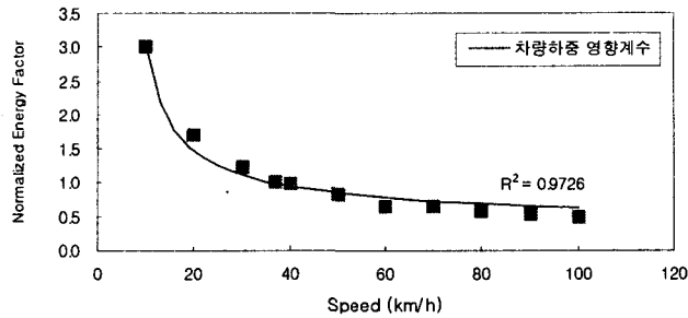
그림 6. 차량속도에 따른 차량하중 영향계수
