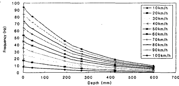
그림 3. 차량 속도에 따른 깊이별 하중주파수
