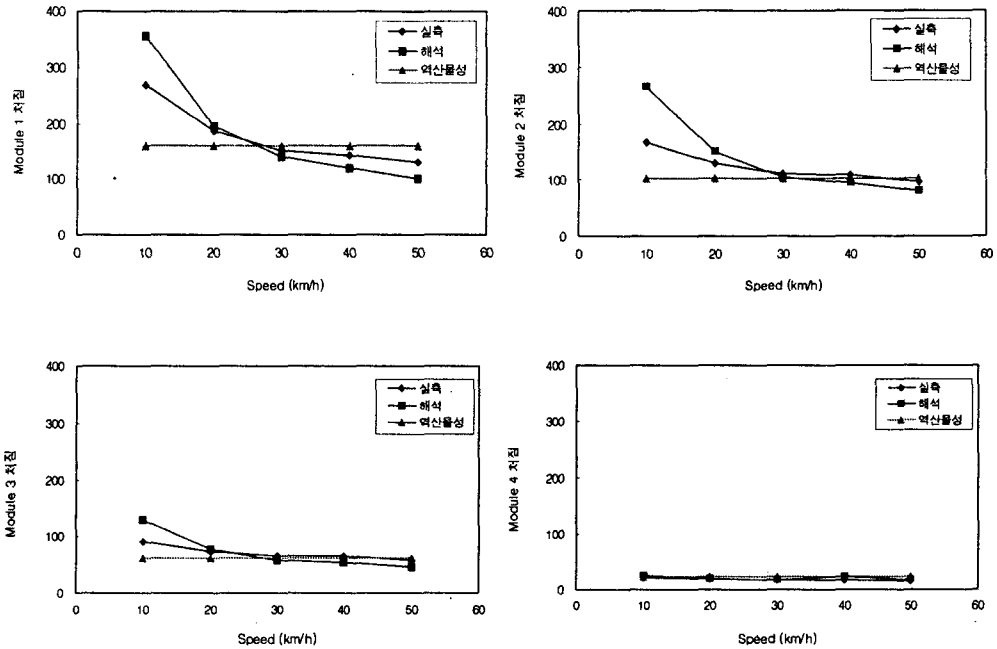
그림 8. 주행속도에 따른 MDD 실측결과의 비교
