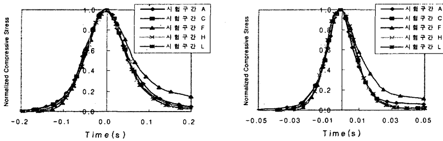
(a) 차량주행속도 8km/h일 경우
