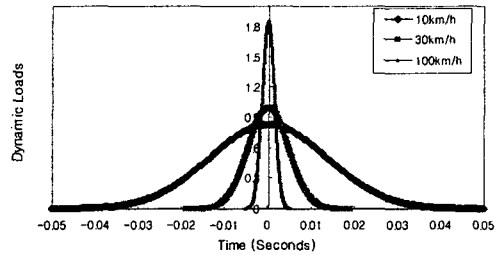
그림 5. 주행차량 속도에 따른 하중곡선 (일례)
