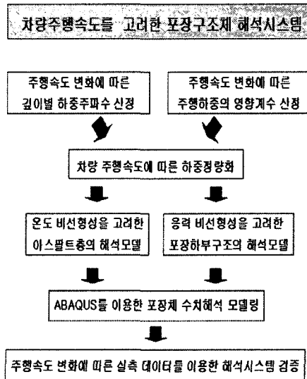
그림 7. 주행차량을 고려한 아스팔트 포장체의 해석시스템 흐름도
