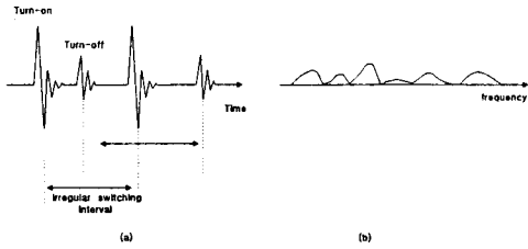
〈그림 3-4〉 RPWM 스위칭노이즈 파형과 스펙트럼 (a) 파형 (b) 스펙트럼
