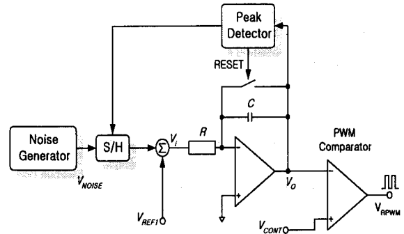
〈그림 3-6〉 RPWM 구성도
