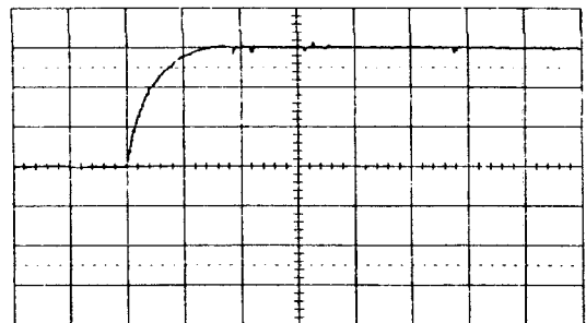
〈그림 4-5〉 RPWM시 출력전압 (Voltage : 100V/div, Time : 50ms/div, 랜덤신호 5%주입)
