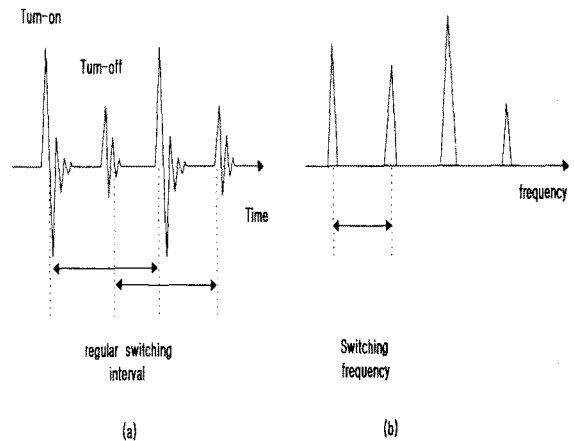
〈그림 3-3〉 PWM 스위칭노이즈 파형과 스펙트럼 (a) 파형 (b) 스펙트럼
