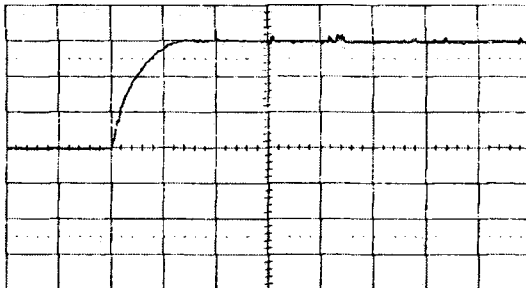
〈그림 4-8〉 반송파 선택회로 출력전압
