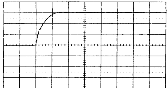
〈그림 4-4〉 PWM시 출력전압 (Voltage : 100V/div, Time : 50ms/div)
