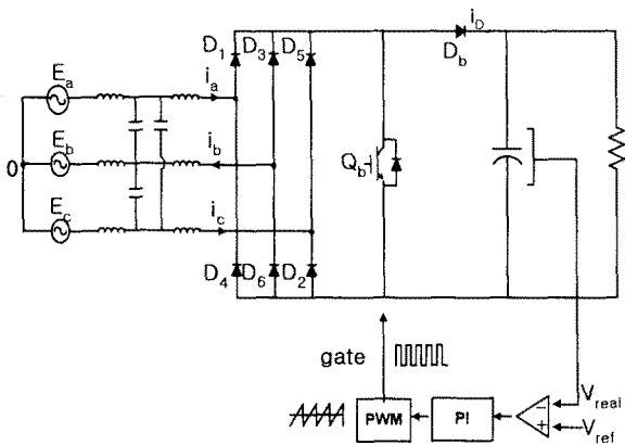
〈그림 3-1〉 단일 스위치 3상 승압형 컨버터
