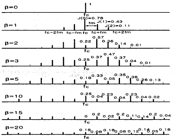
〈그림 3-5〉 \beta 에 따른 이산되는 신호스펙트럼
