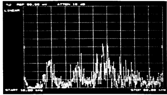
〈그림 4-2〉 RPWM시 스위칭 노이즈전류 (Current : 5mA/div, Frequency Range : 10[kHz] ~ 60[kHz], 랜덤신호 5% 주입)
