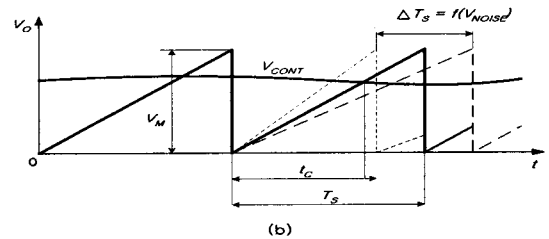
〈그림 3-7〉 RPWM 각부 신호파형 (a) 입력전압 (b) 반송파 발생기의 출력전압
