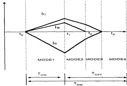
〈그림 3-2〉 한 스위칭 주기 동안의 각 입력 상전류 파형
