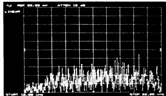
〈그림 4-3〉 RPWM시 스위칭 노이즈전류 (Current : 5mA/div, Frequency Range : 10[kHz] ~ 60[kHz], 랜덤신호 30% 주입)
