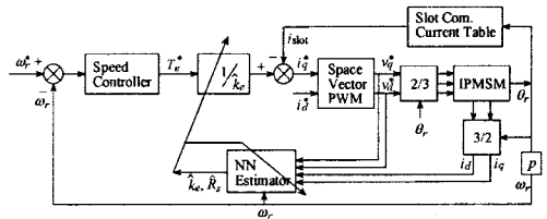
그림 4 혼합 토크리플의 최소화 제어기에 대한 블록도
