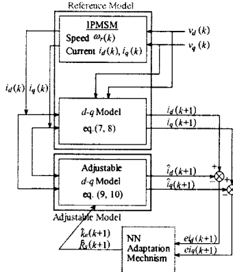
그림 2 토크 정수와 고정자 저항을 위한 MRAS-NN에 의한 추정자
