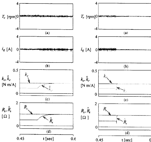
그림 7 PI 제어기에 의한 파라미터 추정특성 그림 8 신경회로망에 의한 파라미터 추정특성
