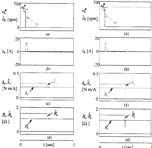
그림 5 PI제어기에 의한 파라미터 응답특성 그림 6 신경회로망에 의한 파라미터 응답특성
