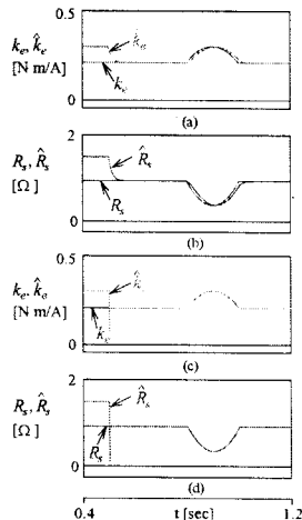
그림 9 토크 정수와 고정자 저항의 추정 특성 비교
