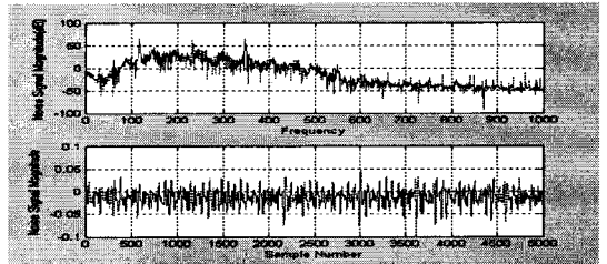
그림 11. 제어전의 FFT 및 소음 파형
