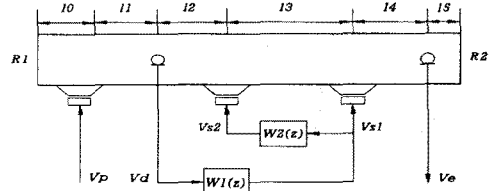
그림 2. 이중극 시스템의 구성도
