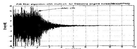
그림 4. 이중극, FXLMS 알고리즘
