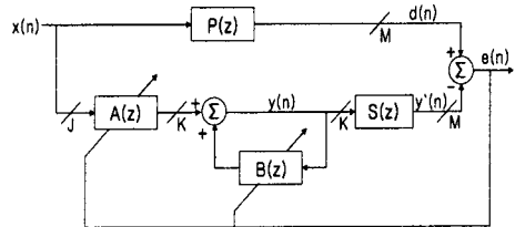
그림 1. 다중채널 순환 LMS 알고리즘의 블록선도
