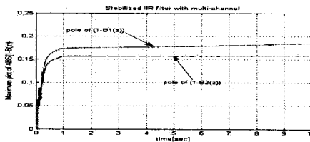
그림 9. 제안된 RLMS의 극점 궤적
