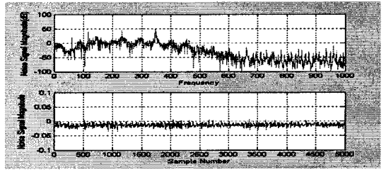
그림 12. 제어후의 FFT 및 소음 파형
