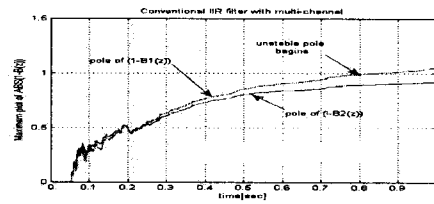
그림 8. 기존의 RLMS의 극점 궤적
