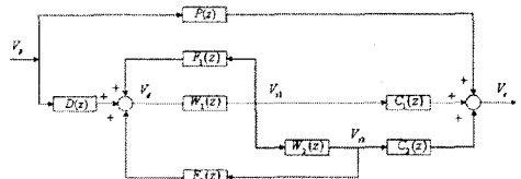
그림 3. 이중극 시스템의 블록선도
