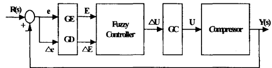
그림 3. Fuzzy 제어기
