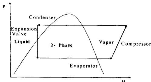
그림 2. 에어컨 사이클 및 모리엘 선도(p-h선도)
