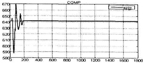
그림 5. 이산형 lookup_table 방식의 저압
