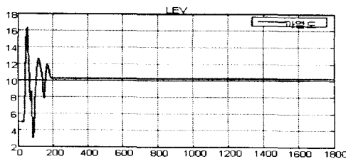
그림 7. 이산형 lookup_table 방식의 과열도
